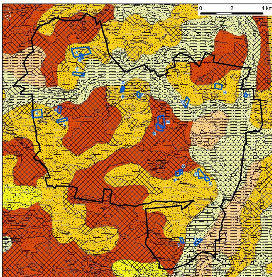
Ryc. 4. Budowa geologiczna i litogenetyczna gminy Kąkolewnica
